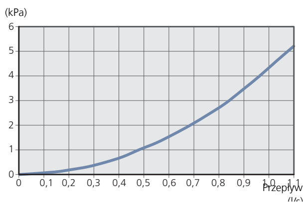
Spadek ciśnienia
