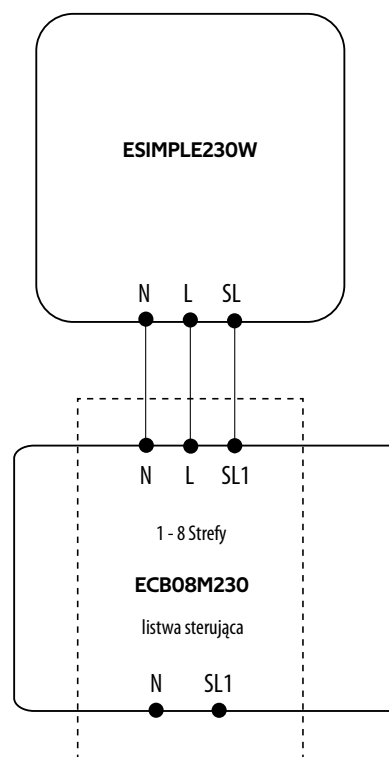
b) Schematy podłączenia do listwy sterującej
